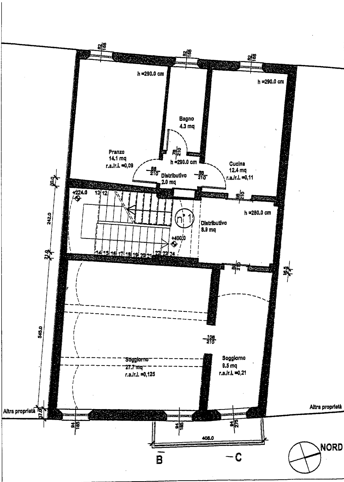
PIANO PRIMO
