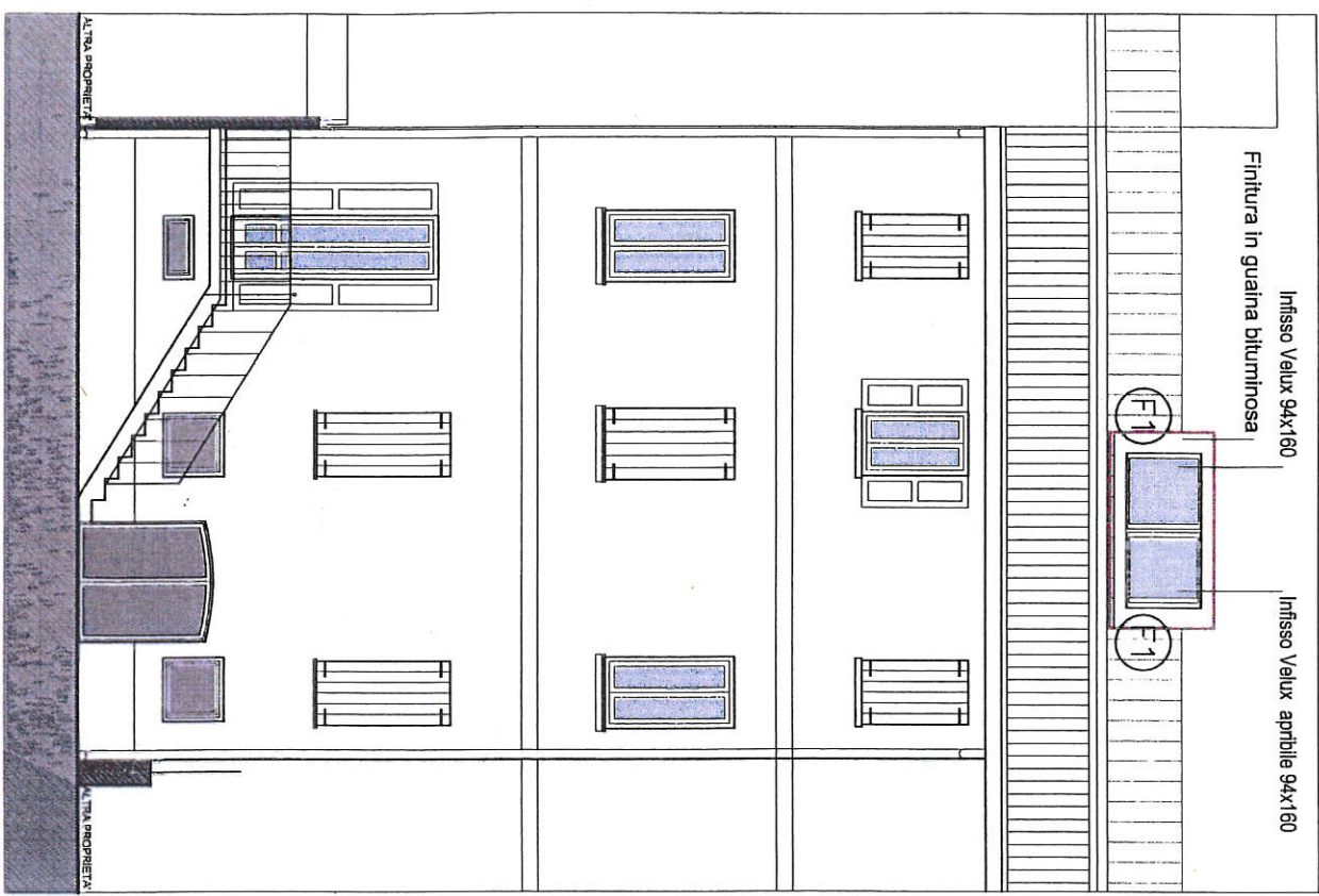
PROSPETTO SUL CORTILE INTERNO
